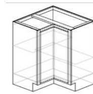
Easy Reach with Hinged Door (BER3636)
